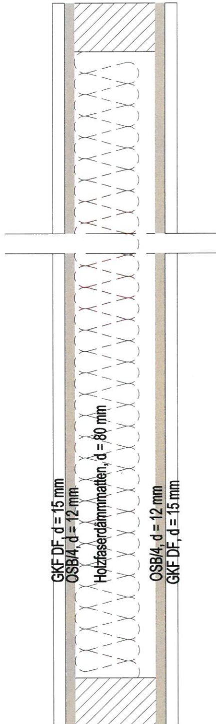
Abbildung A1.2 Vertikalschnitt durch die Konstruktion
