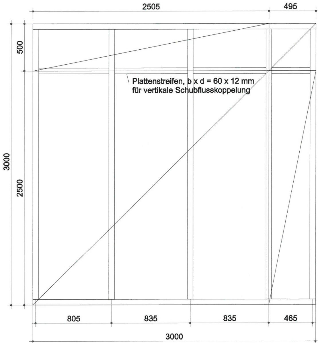
Abbildung A1.1 Anordnung der Tragkonstruktion und der Bekleidung/Bepankung aus OSB/4-Platten
