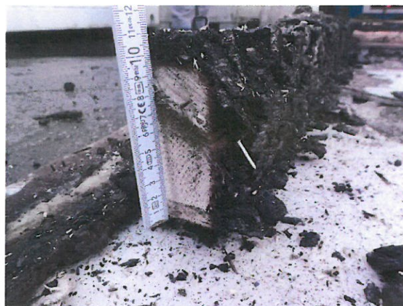
Bild A6.8 Restquerschnitt Ständer 1.
