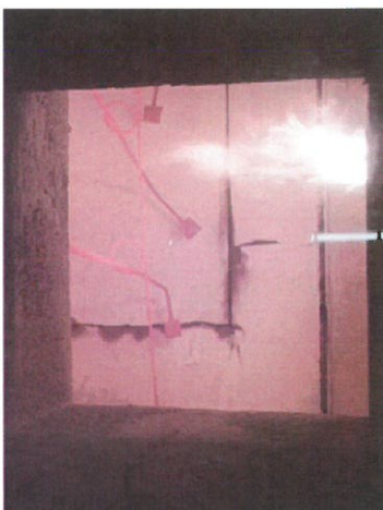
Bild A6.5 Prüfminute 32: Fugen der Feuerschutzplatten ca. 3 mm geöffnet, Schwarzer Fugengrund.
