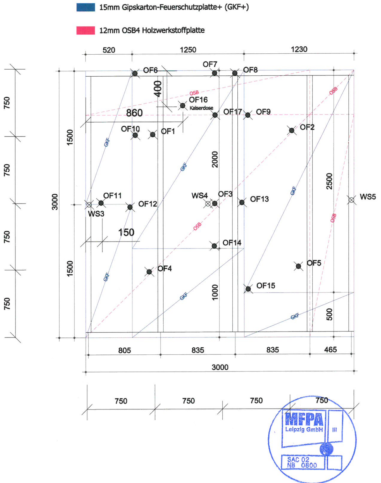
Abbildung A2.1 Anordnung der Messstellen auf der Prüfkörperoberfläche (feuerabgewandte Seite)
